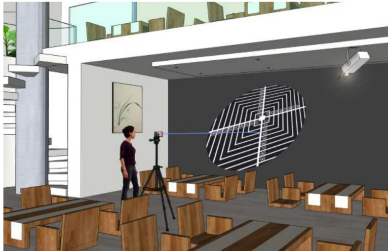
Abb. 2: Das projizierte Messgobo wird fotografiert. Dabei muss die Kamera rechtwinklig zur Projektions-fläche ausgerichtet sein, dargestellt durch die blaue Linie.
